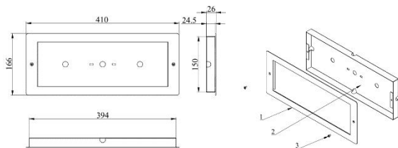
壁挂灯具暗装示意图（YMH-BZ07 专用预埋盒）
