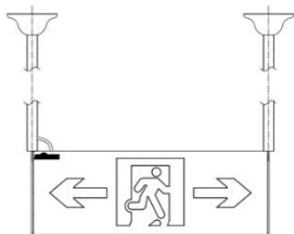
吊装灯具安装示意图
